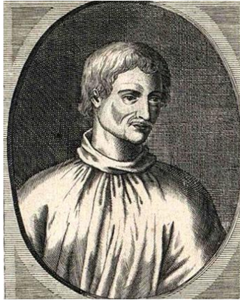
Giordano Bruno
