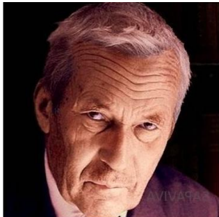
Andreï Kolmogorov
