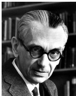
Kurt Gödel
