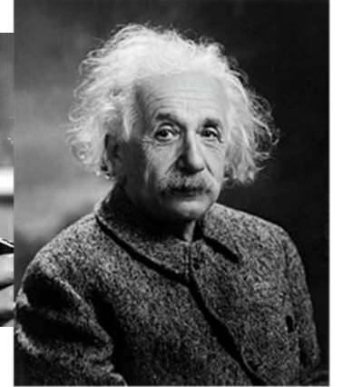
Albert Einstein
