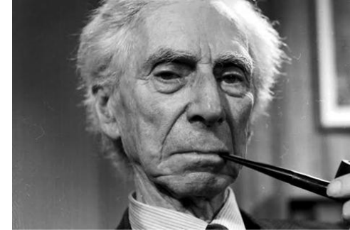
Bertrand Russell
