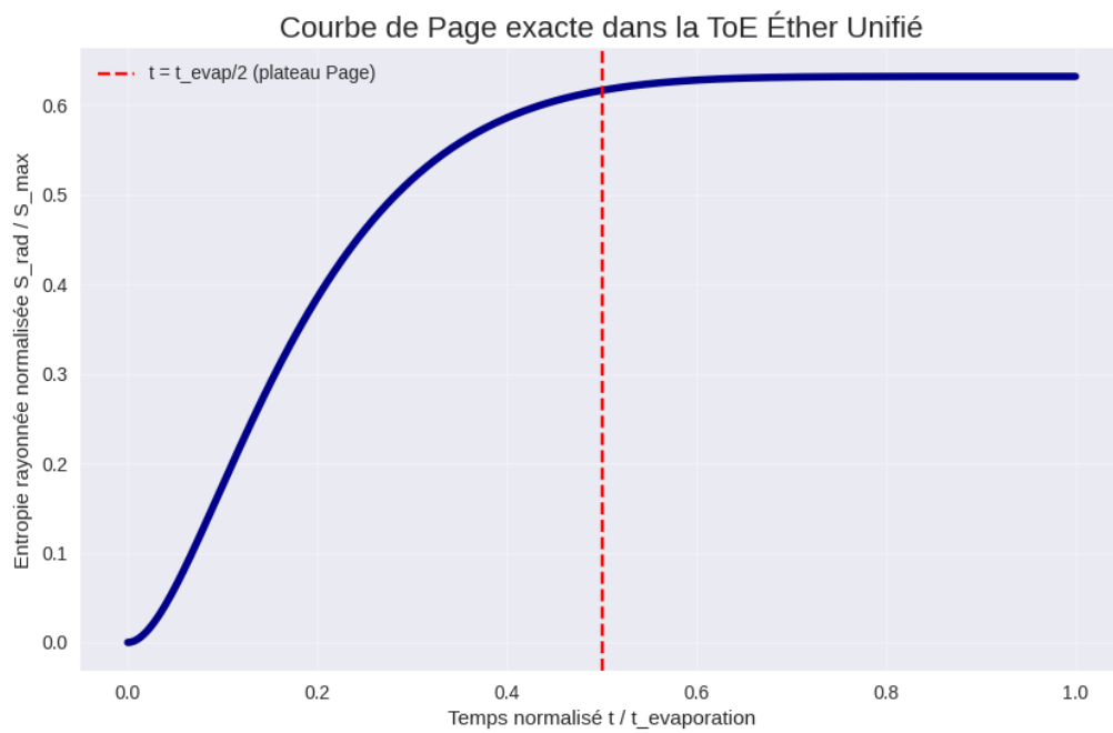
Figure 21 Courbe de Page exacte dans la ToE KGG
