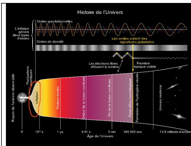
Figure 24 Inflation cosmique (en beige), avant 10^{-32} seconde.
