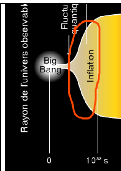
Figure 25 Inflation cosmique détail
