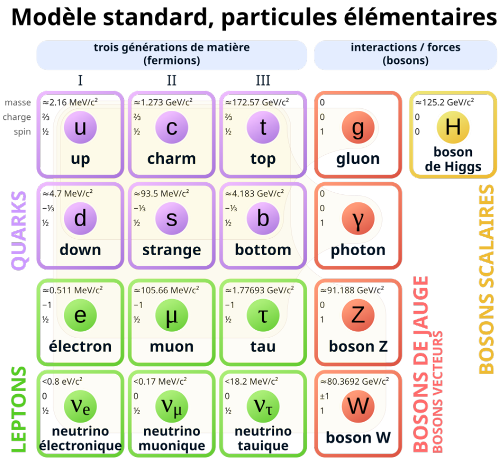
Figure 26 Modèle standard des particules élémentaires avec les trois générations de fermions (trois premières colonnes), les bosons de jauge (quatrième colonne) et le boson de Higgs.
