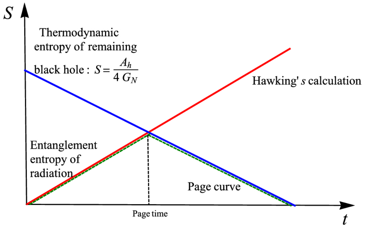
Figure 22 La courbe de Page, représentée par la ligne pointillée verte, pour l'évaporation du trou noir compatible avec l'évolution de l'unitarité.
