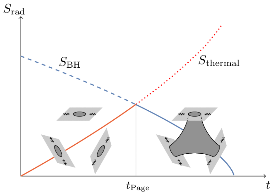
Figure 23 La transition entre les topologies déconnectées et connectées dans l'intégrale de chemin gravitationnel euclidien donne lieu à une courbe de Page pour l'entropie du rayonnement de Hawking.
